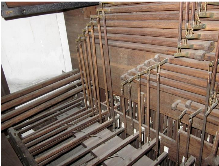
Een wellenbord uit het midden van de zeventiende eeuw, hier voor de verbinding tussen pedaal en manuaal (Amsterdam, Nieuwe Kerk, transeptorgel).
